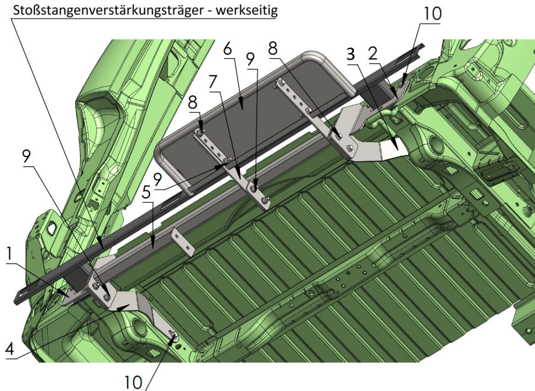
Rys 1.2 Widok montażowy przykręconego zespołu podestu do ramy pojazdu. Montageansicht der am Fahrzeugrahmen verschraubten Podestbaugruppe.
