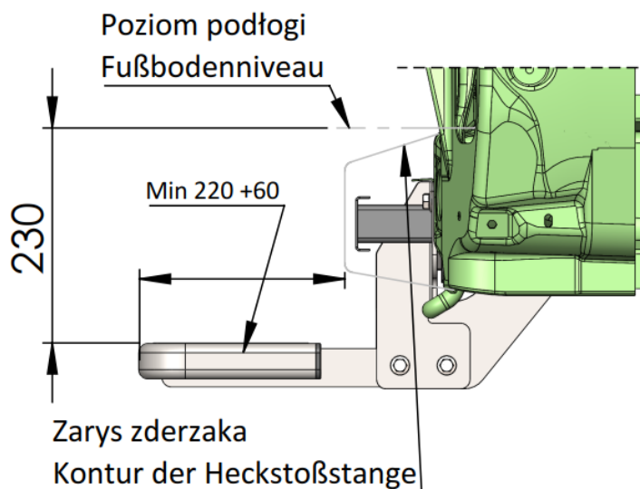
Rys 1.1 Prawidłowe wymiary po montażu podestu do pojazdu. Korrekte Abmessungen nach der Montage der Plattform am Fahrzeug.
