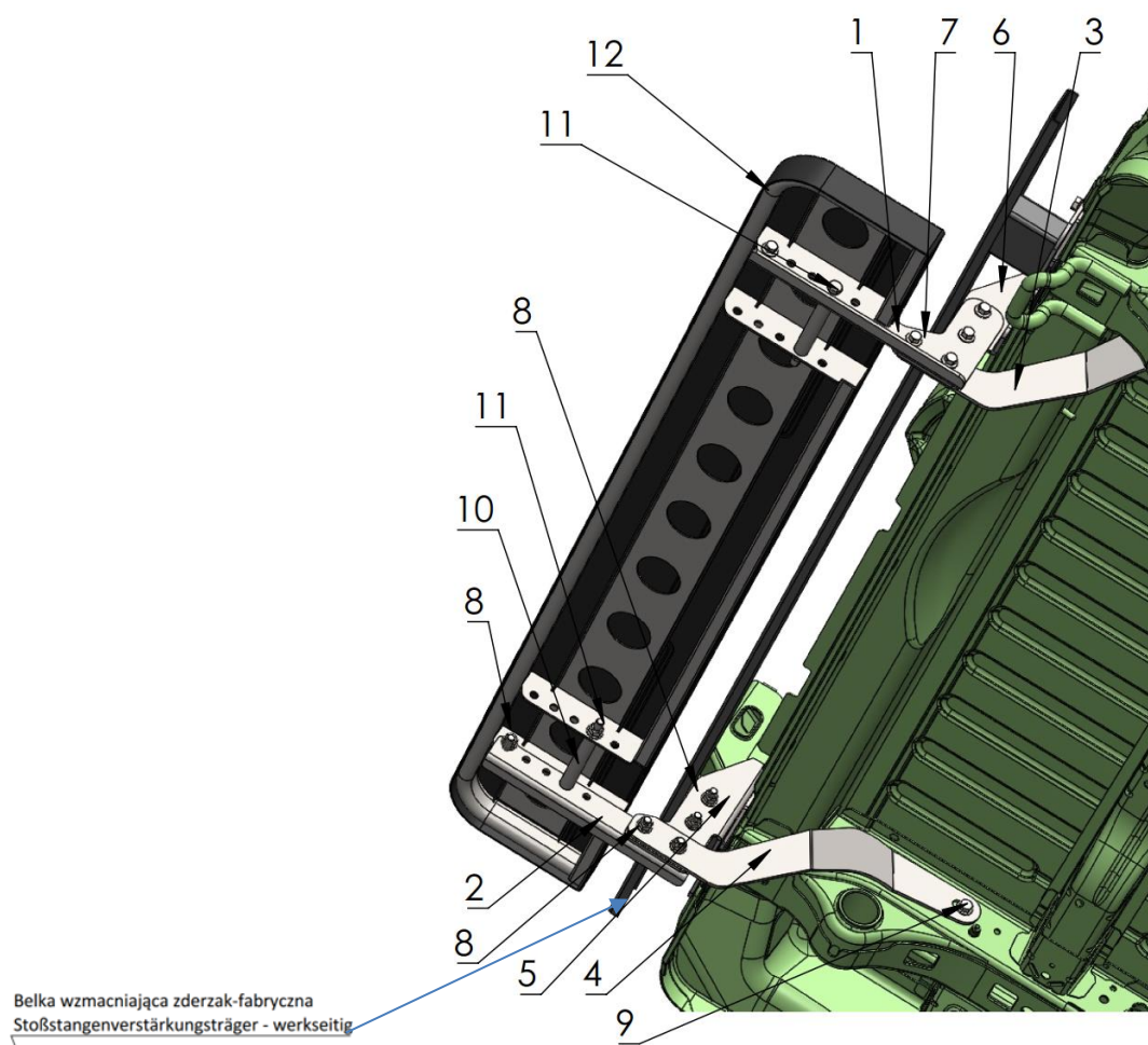
Rys 1.2 Widok montażowy przykręconego zespołu podestu do ramy pojazdu. Montageansicht der am Fahrzeugrahmen verschraubten Podestbaugruppe.
