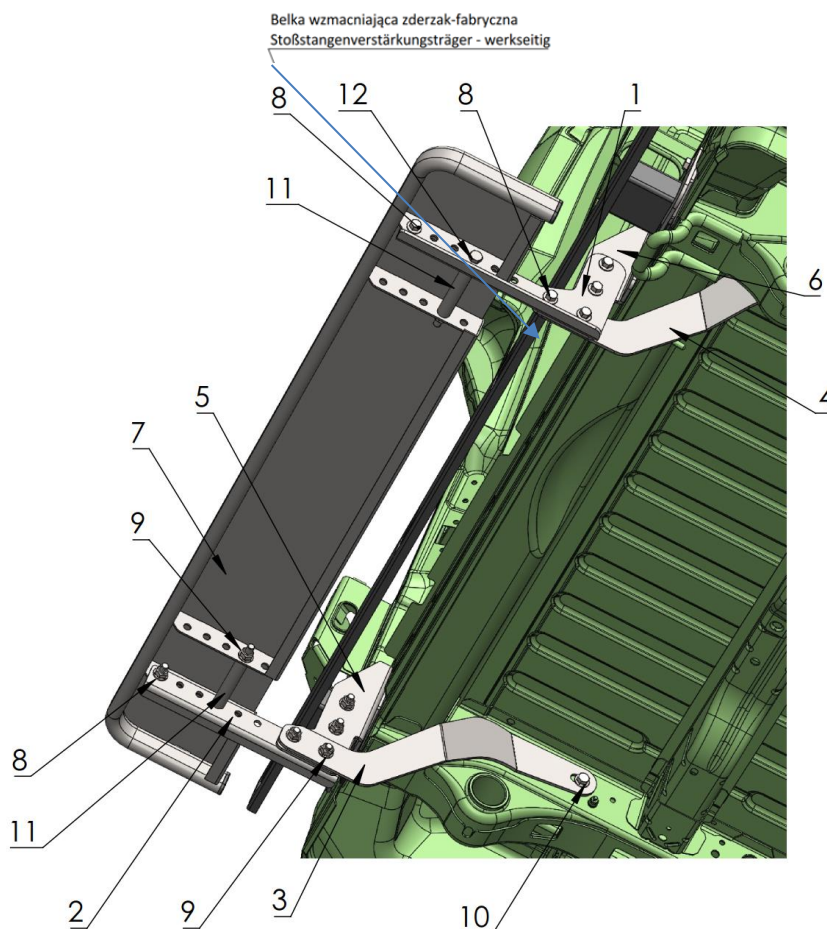
Rys 1.2 Widok montażowy przykręconego zespołu podestu do ramy pojazdu. Montageansicht der am Fahrzeugrahmen verschraubten Podestbaugruppe.
