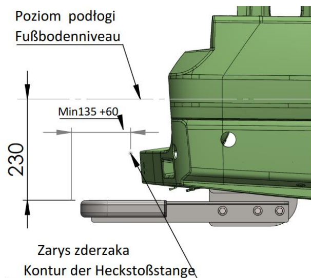
Rys 1.1 Prawidłowe wymiary po montażu podestu do pojazdu. Korrekte Abmessungen nach der Montage der Plattform am Fahrzeug.
