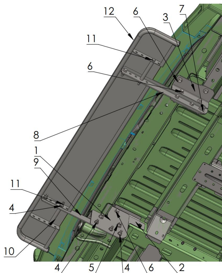
Rys 1.2 Widok montażowy przykręconego zespołu podestu do ramy pojazdu Montageansicht der am Fahrzeugrahmen verschraubten Podestbaugruppe
